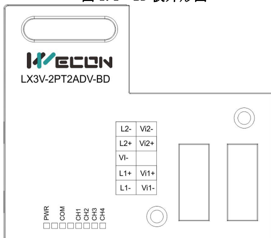
图 1.1 BD 板外形图
