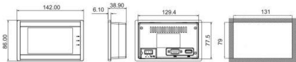
PI3043ie-T 安装尺寸图
