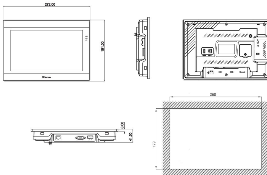
PI3102ig/ PI3102ig-C 安装尺寸图
