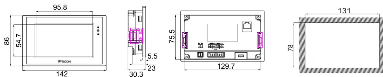
PI3043ie / PI3043ie-N 安装尺寸图
