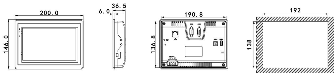
PI3070i-A 安装尺寸图
