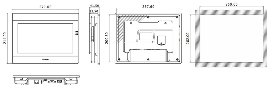
IN1101 安装尺寸图
