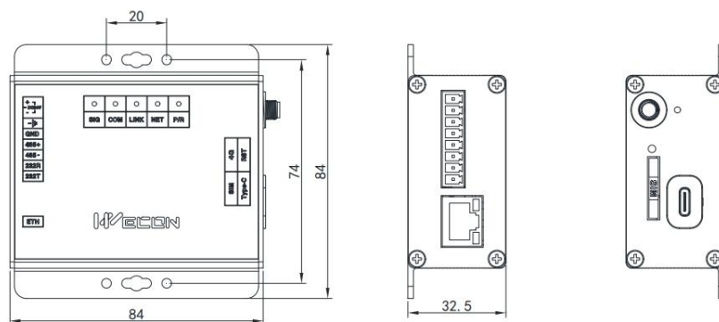
RL-WF/RL-G 安装尺寸图
