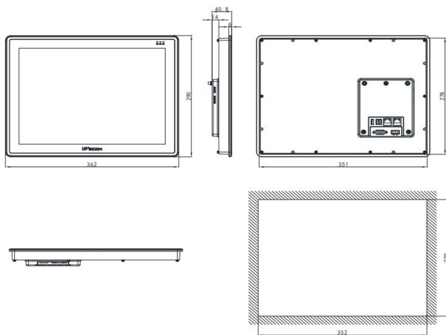
PI8151ig(N) 安装尺寸图
