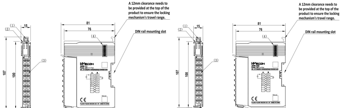
(1) DIN rail clip; (2) I/O indicator; (3) I/O terminal; (4) Right expansion interface
