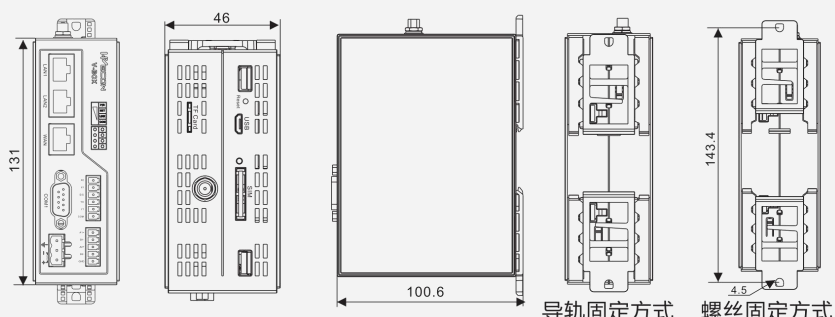
V-BOX H-00/H-WF/H-4G/H-AG 安装尺寸图
