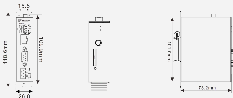
RE-00 / RE-4G 安装尺寸图
